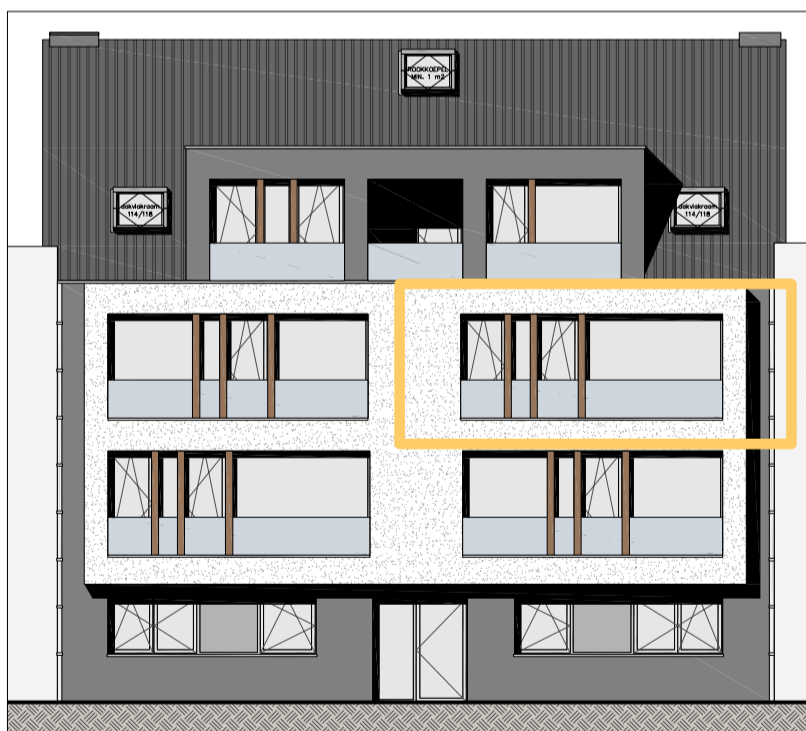
VOORGEVEL
