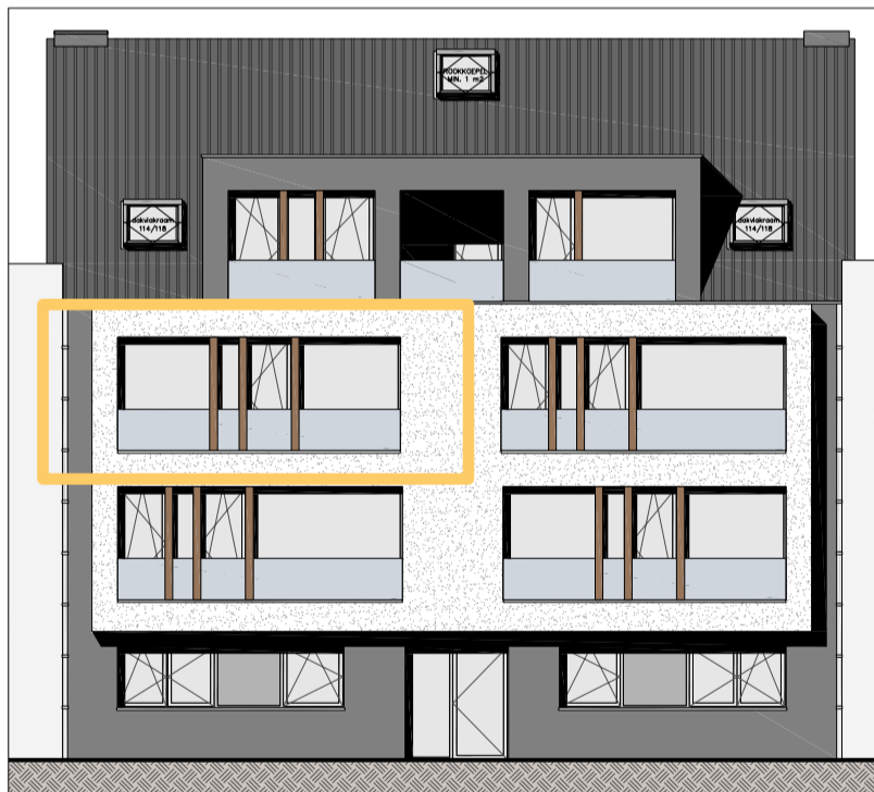
VOORGEVEL
